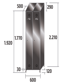
SV-30/2 INOX COD: 83902 49kg · 0,69m 3
