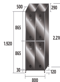
SV-40/2 INOX COD: 84902 59kg · 0,76m 3
